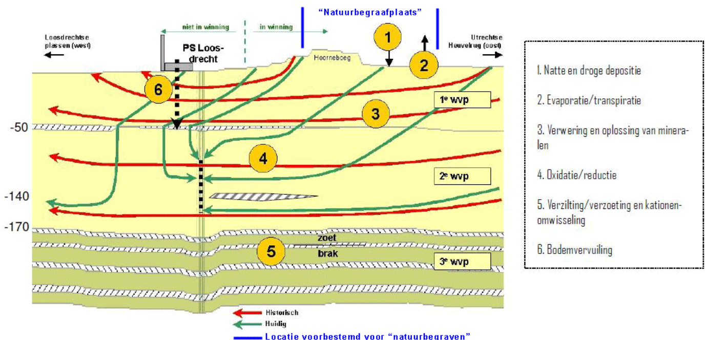
Figuur 1-7 Schematisch beeld van de grondwaterstroming (historisch en huidig) met een zwarte stippellijn voor de invloed van dichtheidsstroming
